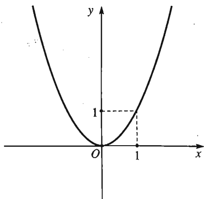
Đồ thị hàm số y = f(x)
